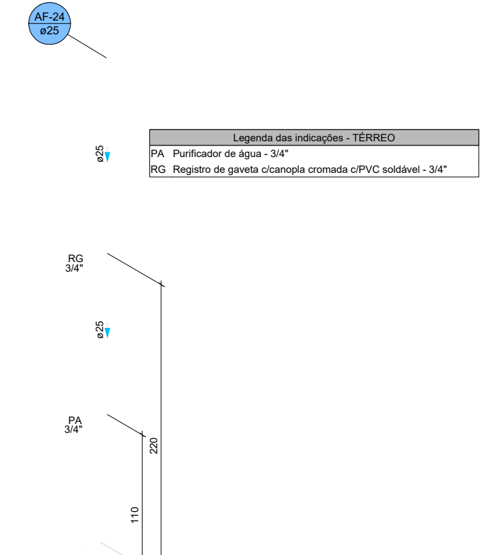
DETALHE HID-24 1:25
