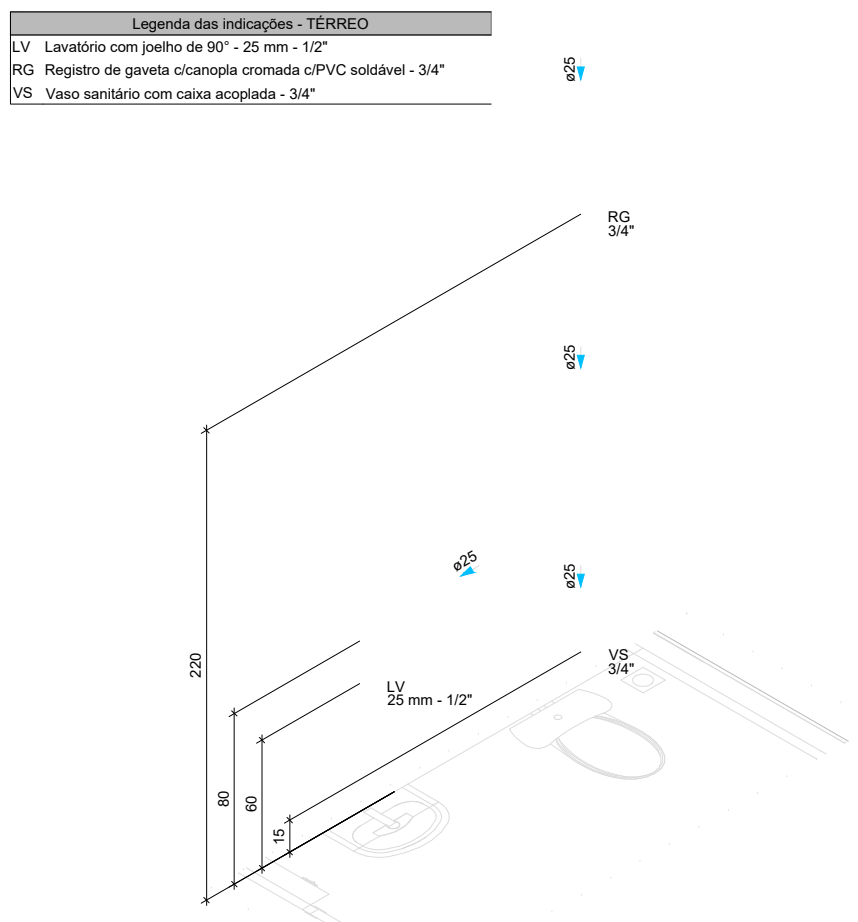
DETALHE HID-22 1:25
