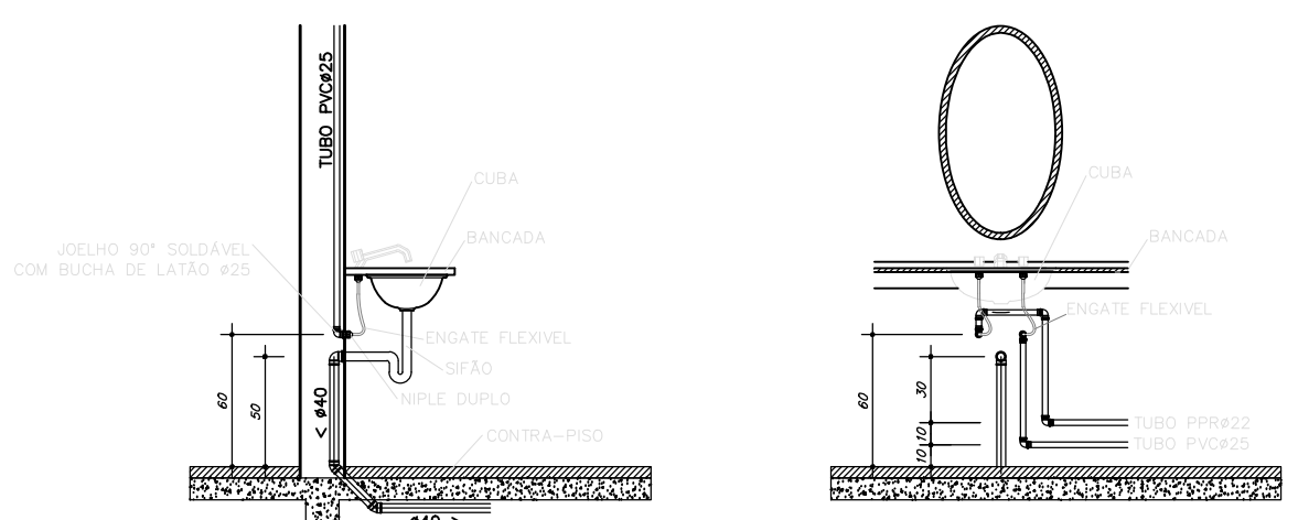
VISTA LATERAL DA LIGAÇÃO DE ÁGUA/ESGOTO Sem Escala VISTA FRONTAL DA LIGAÇÃO DE ÁGUA/ESGOTO Sem Escala
