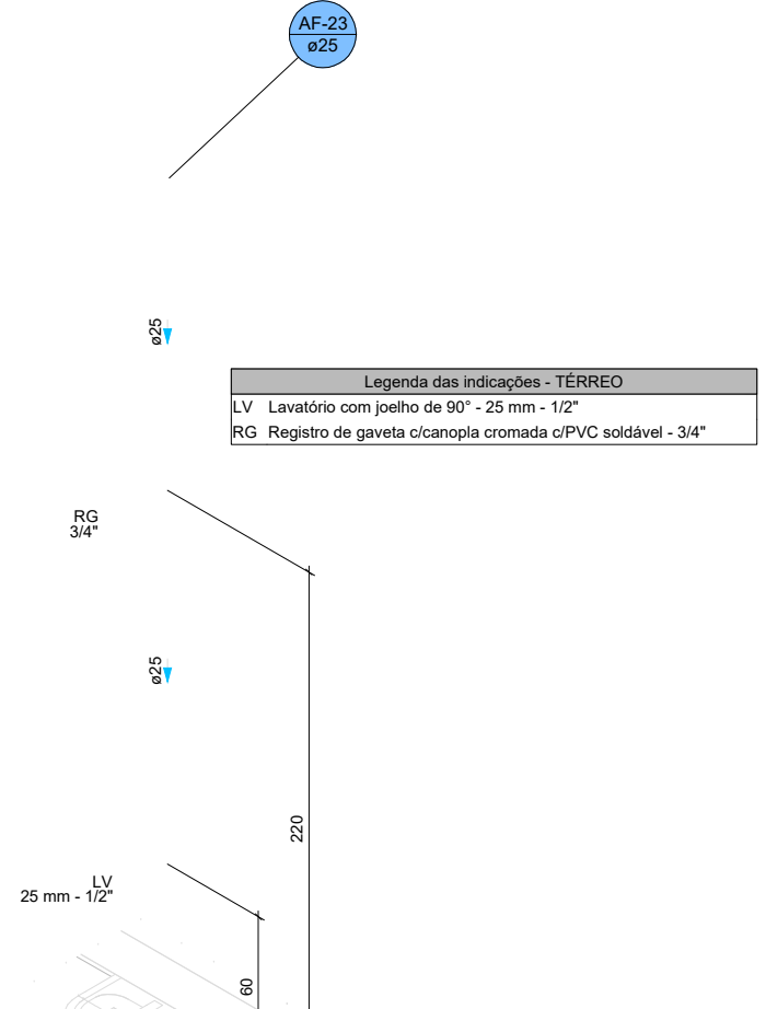
DETALHE HID-23 1:25
