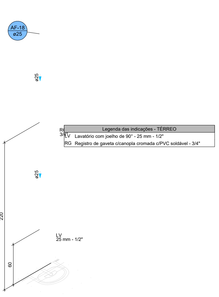
DETALHE HID-18 1:25
