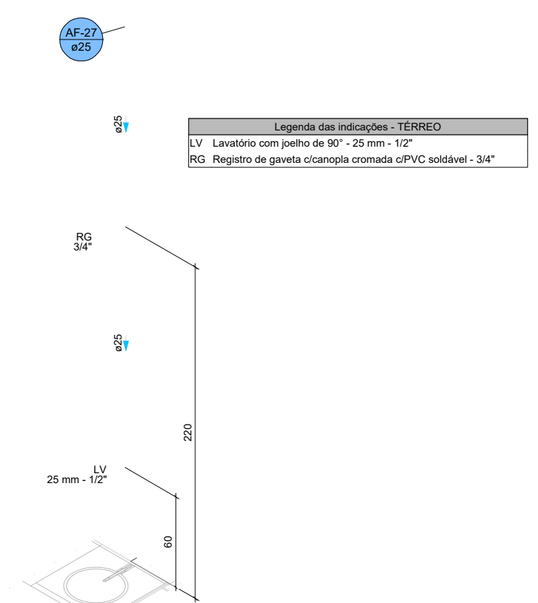
DETALHE HID-26 1:25
