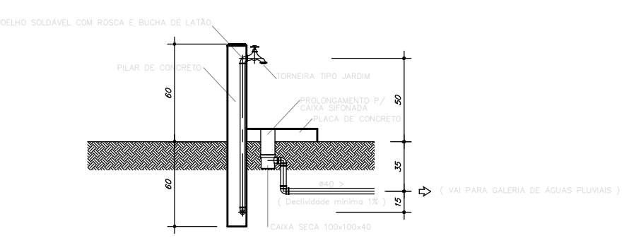
VISTA LATERAL PUNTO DE ÁGUA EXTERNO Sem Escala
