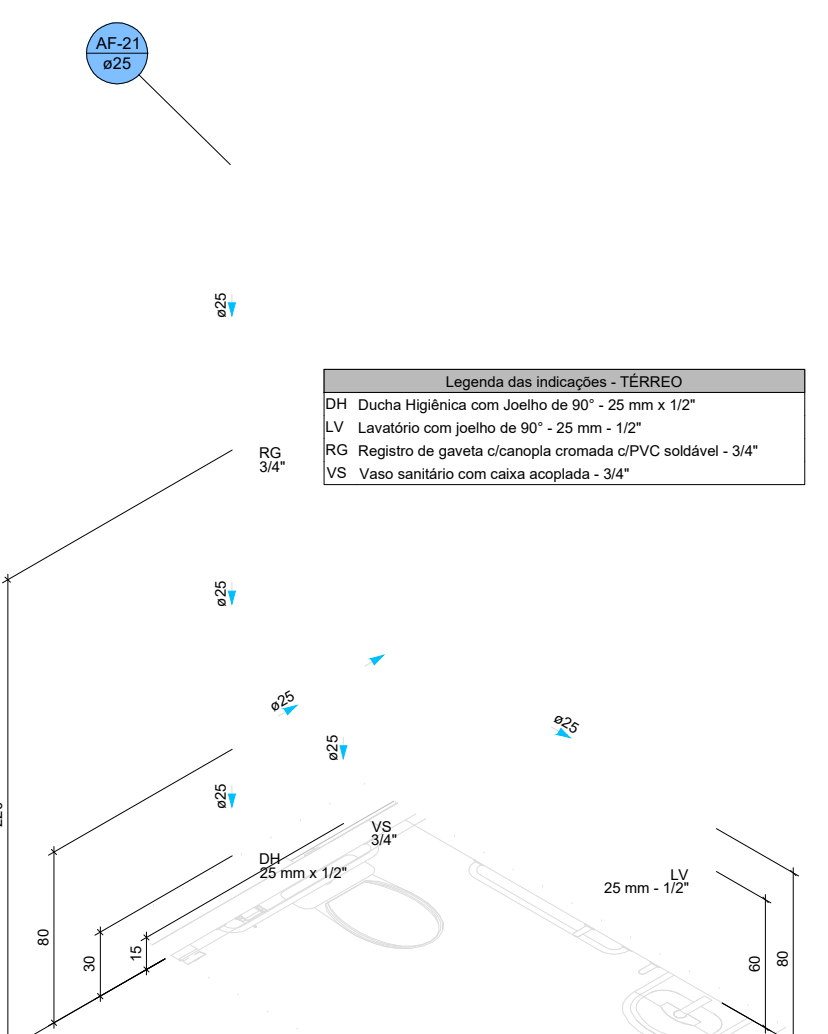
DETALHE HID-16 1:25
