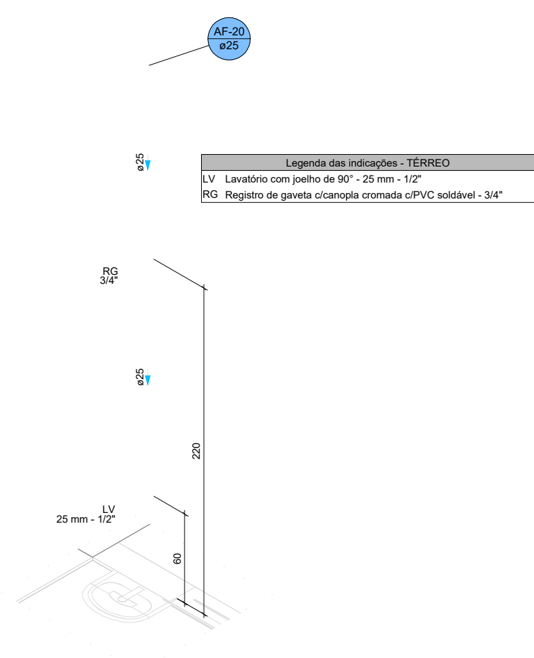
DETALHE HID-19 1:25
