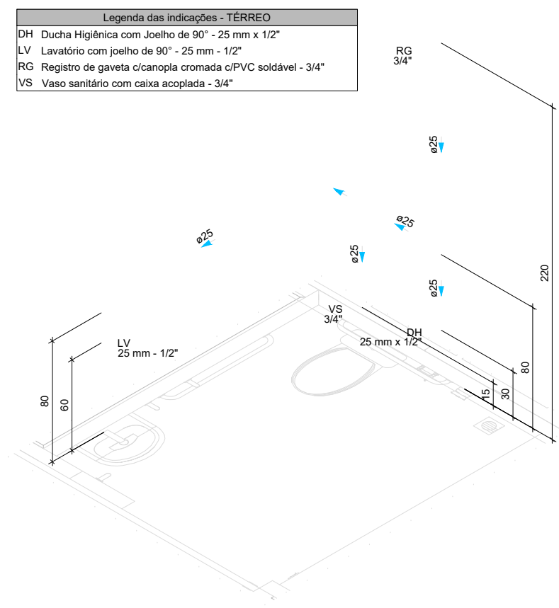
DETALHE HID-16 1:25
