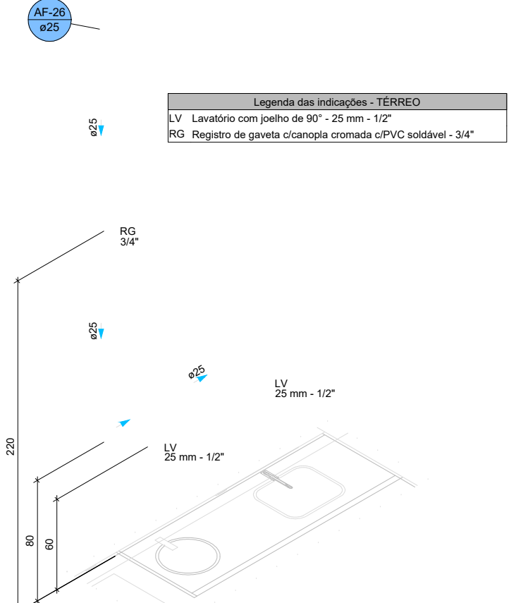
DETALHE HID-25 1:25
