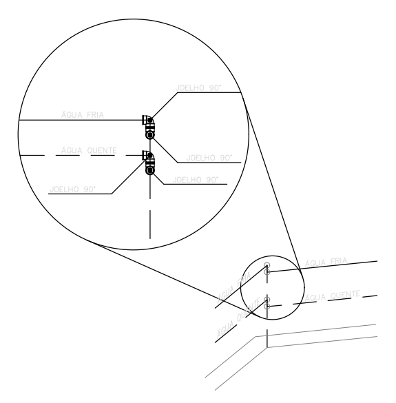
DETALHE PARA CANTOS DE PAREDE Escala 1/25
