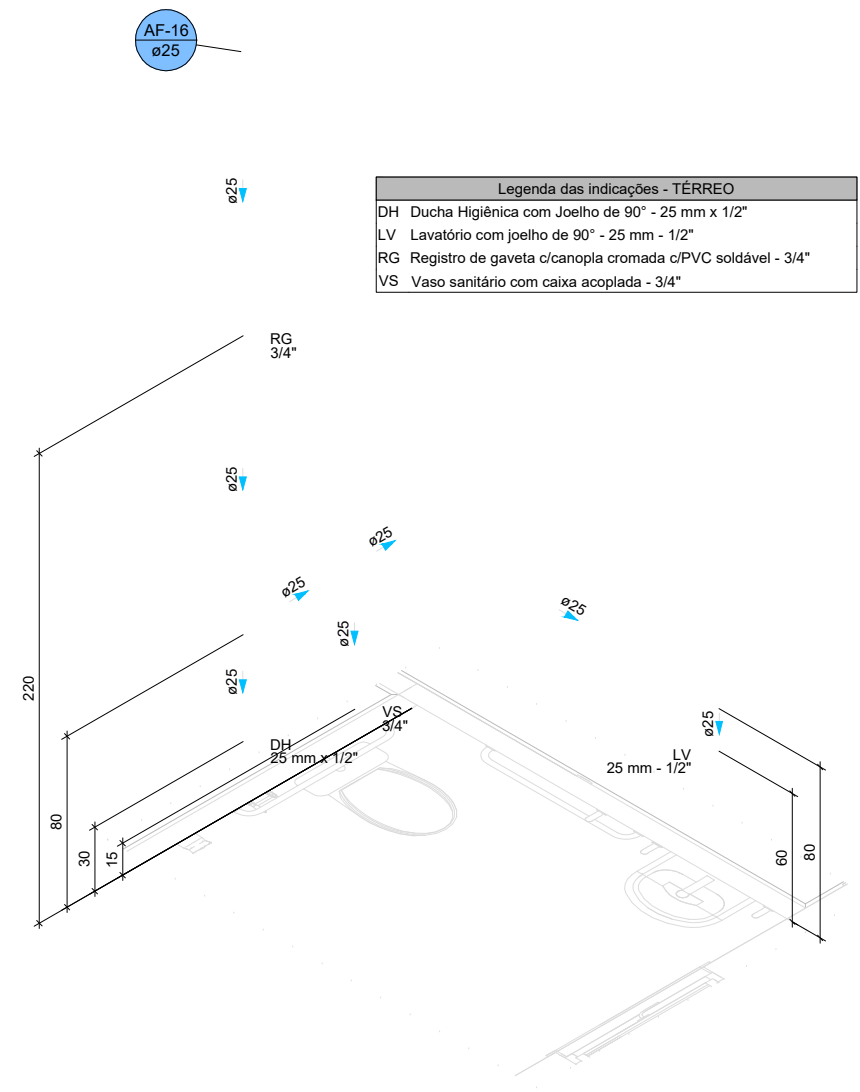
DETALHE HID-17 1:25
